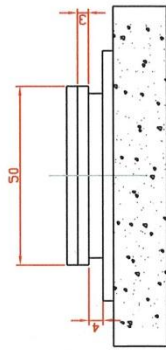
vooraanzicht
